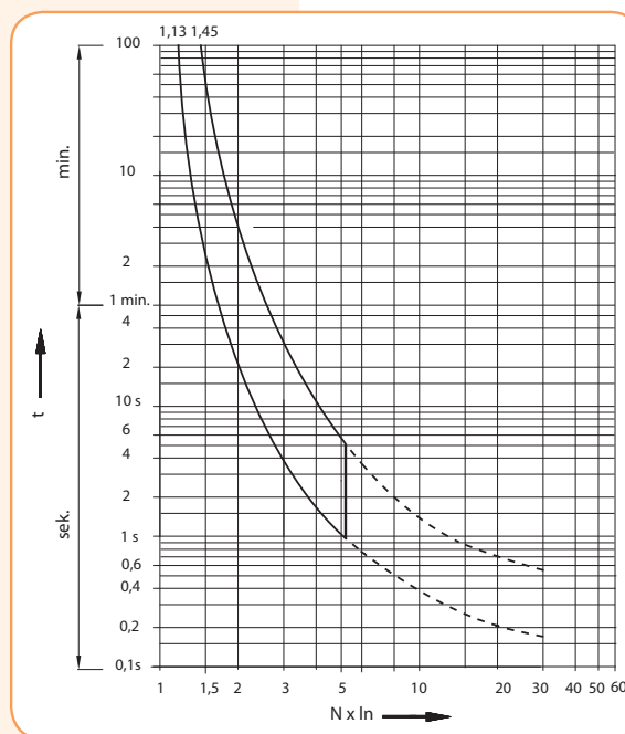
Charakterystyka czasowo-prądowa t-I ogranicznika mocy ETIMAT T
