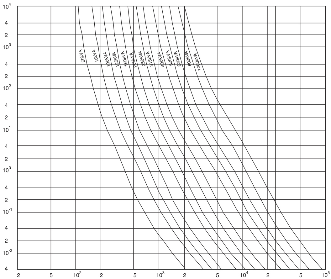
Charakterystyki czasowo - prądowe (rzeczywiste) wkładek topikowych o charakterystyce gTr - 400V
