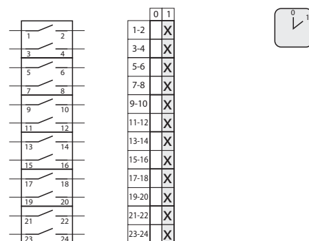
7.8220 Rozł cznik 0-1 (13 - biegunowy)
