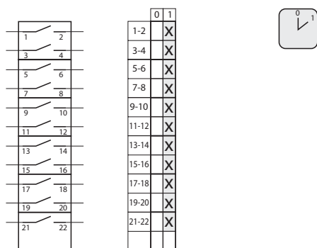
6.8210 Rozł cznik 0-1 (11 - biegunowy)
