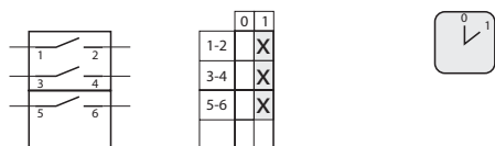
2.423 Rozł cznik 0-1 (3 - biegunowy)
