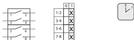
3.8220 Rozł cznik 0-1 (5 - biegunowy)
