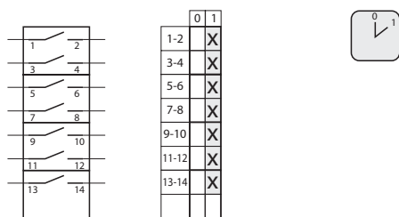
4.824 Rozł cznik 0-1 (8 - biegunowy)
