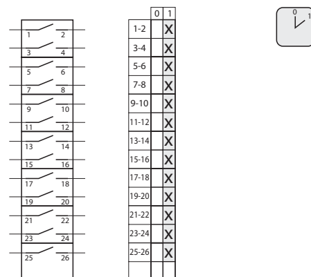
7.822 Rozł cznik 0-1 (14 - biegunowy)
