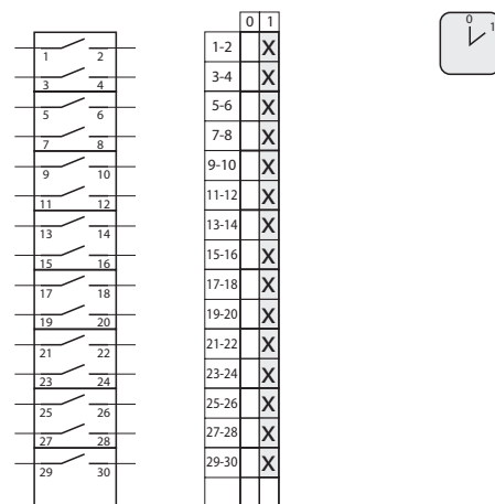
8.8270 Rozł cznik 0-1 (15 - biegunowy)
