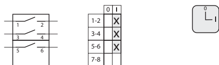
2.4226 Rozł cznik 0-1 (4 - biegunowy)
