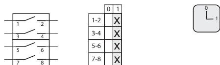
2.8210 Rozł cznik 0-1 (4 - biegunowy)
