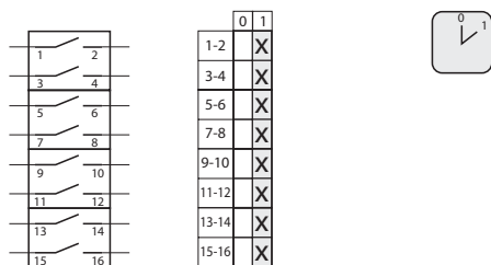
5.8220 Rozł cznik 0-1 (9 - biegunowy)
