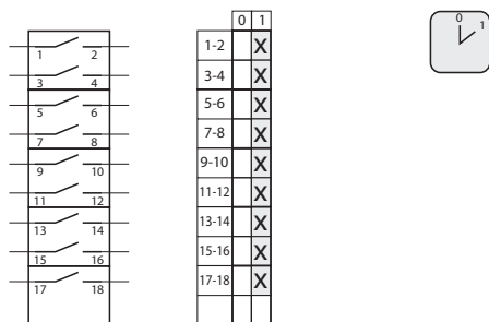
5.822 Rozł cznik 0-1 (10 - biegunowy)
