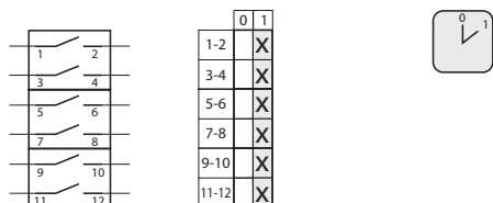
3.8210 Rozł cznik 0-1 (6 - biegunowy)
